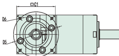
輸入端 Input
