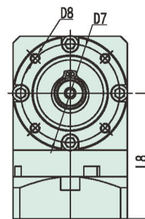
輸出端 Output
