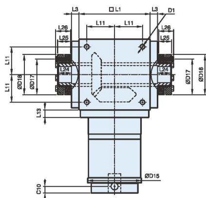
外形尺寸圖 Dimensions:
