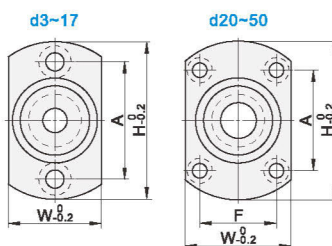
Opposite Edge Flange Type
